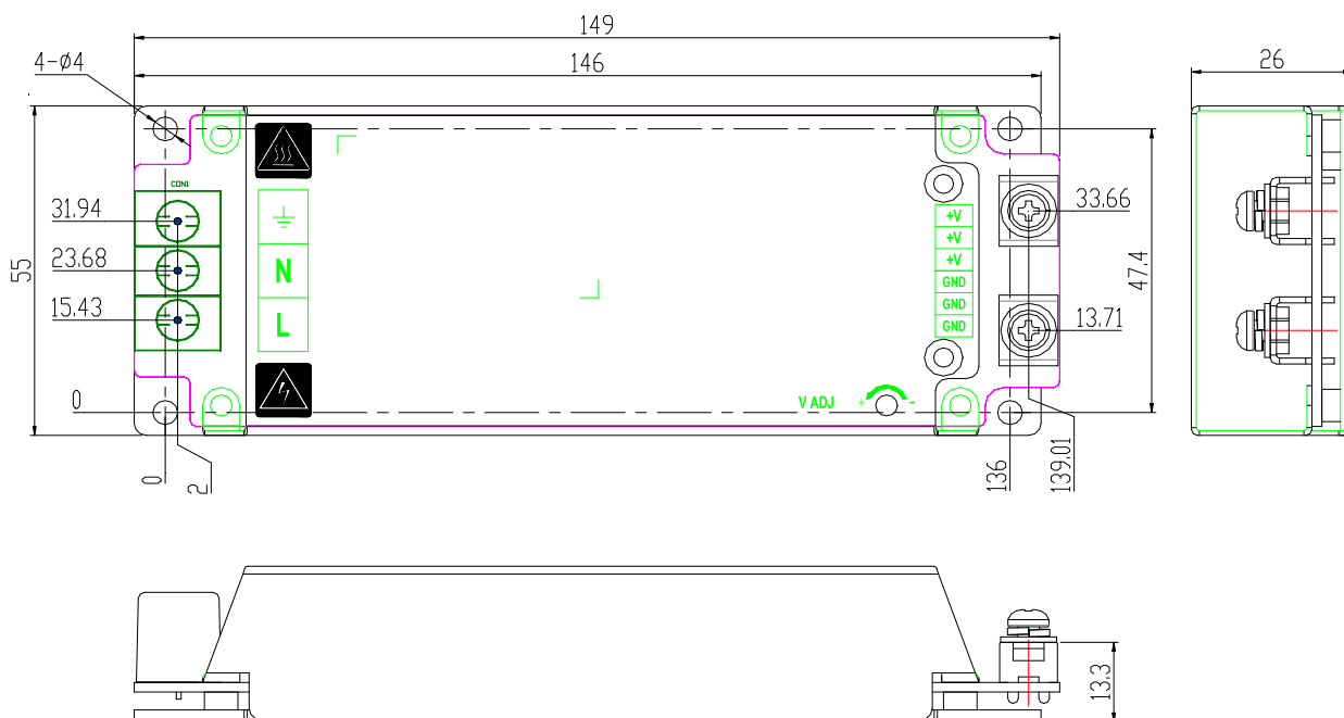
输入、输出端子定义及安装扭力
